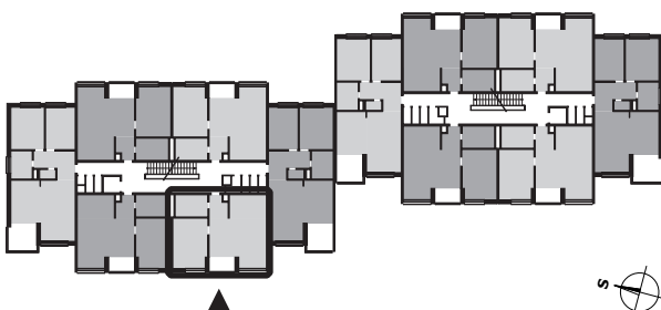
Pôdorys
